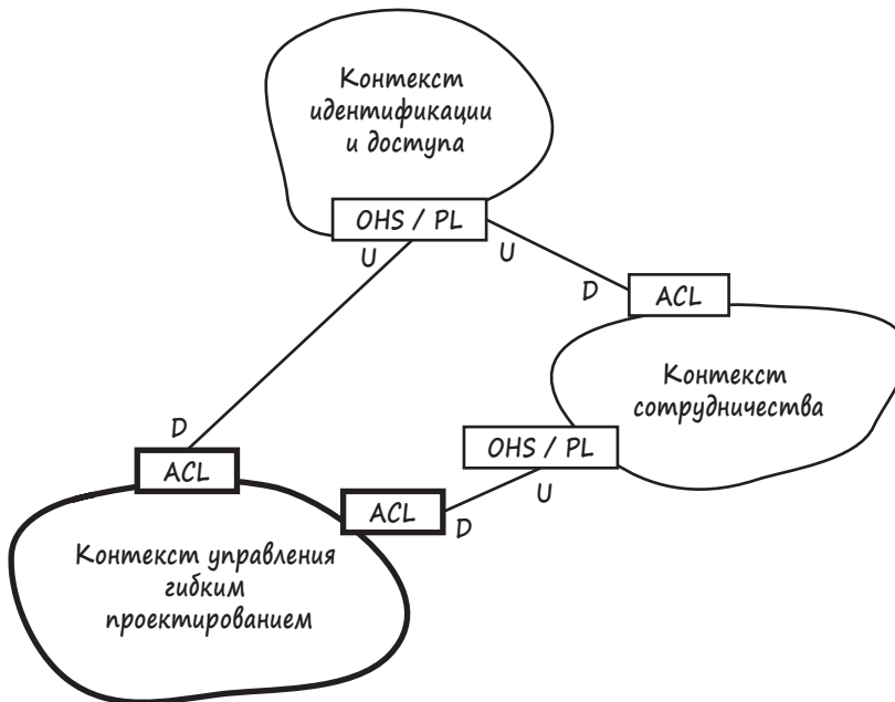
Рис. 3.5. Текущее СМЫСЛОВОЕ ЯДРО обозначено сплошной линией и точками интеграции. СЛУЖЕБНАЯ ПОДОВАСТЬ CollabOvation и НЕСПЕЦИАЛИЗИРОВАННАЯ ПОДОВАСТЬ IdOvation являются нижестоящими
