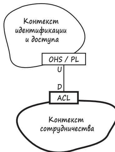
Рис. 3.4. Исходное СМЫСЛОВОЕ ЯДРО обозначено сплошной линией и точками интеграции. В данном случае система IdOvation служит НЕСПЕЦИАЛИЗИРОВАННОЙ ПОДОБЛАСТЬЮ по отношению к нижестоящей системе CollabOvation
