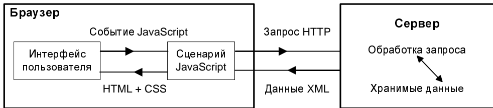
Рис. 1.2. AJAX-модель Web-приложения
